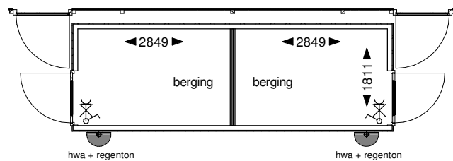
Begane grond
